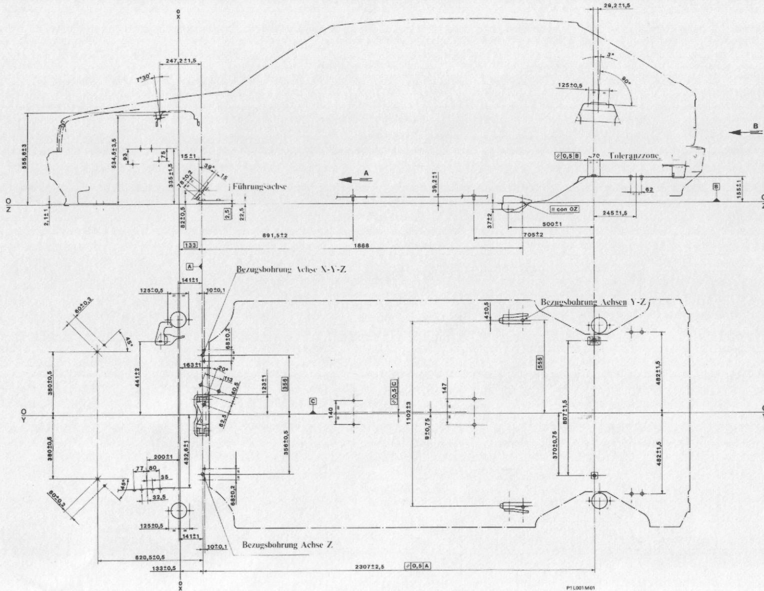
SCHEMA ZUR KONTROLLE DES KAROSSERIEBODENS
